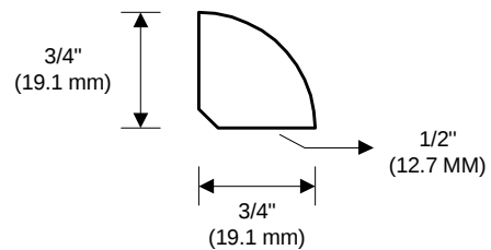
QUARTER ROUND QUART DE ROND
