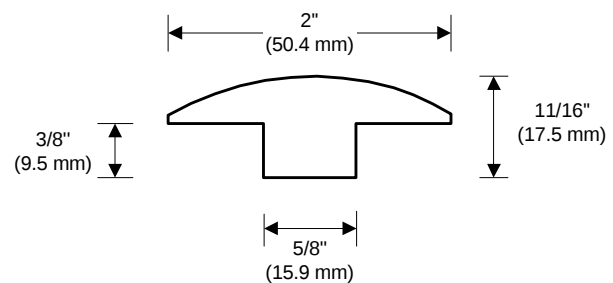
T-MOLDING (SOLID + ENGINEERED FLOOR) MOULURE EN "T" (PLANCHER MASSIF + LAMINÉ)
