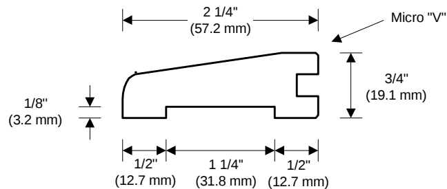
REDUCER (SOLID FLOOR) RÉDUCTEUR (PLANCHER MASSIF)
